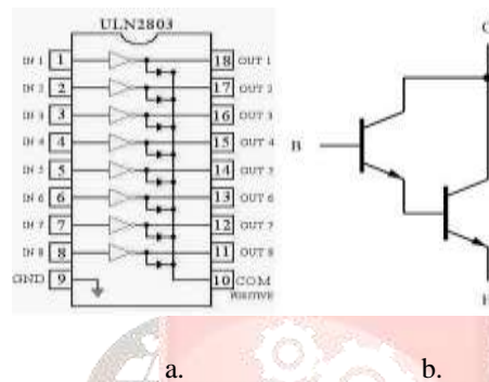
Fig -4: a. ULN 2803; b. Darlington Pair
