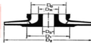
Fig.4: Impeller
